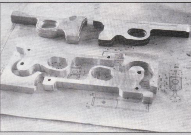
◁ L'évolution de la fabrication des carcasses. D'abord tirées d'un bloc moulé (en haut), elles sont maintenant taillées dans la masse, par paires (en bas).
